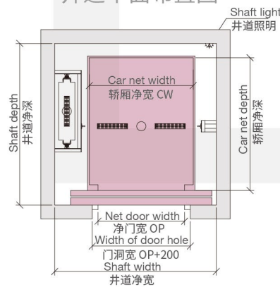
Shaft plane layout 井道平面布置图
